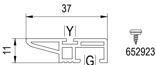
100253 Interlock
